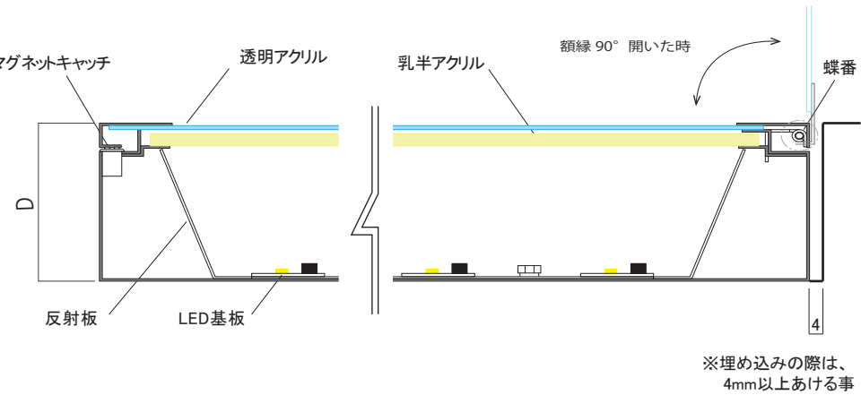
□本体構造断面図 (上図 A-A)
