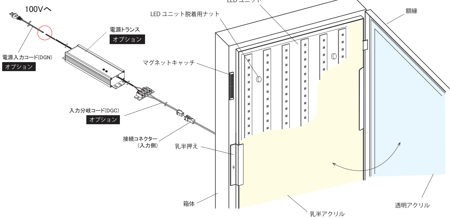
□本体構造図
