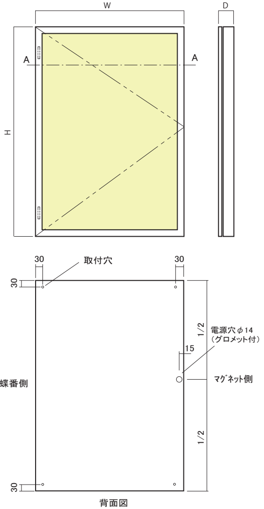
□本体外形図
