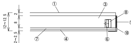
・A-A 断面
