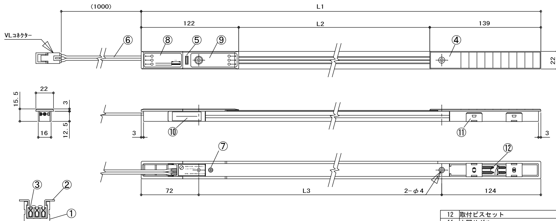
A-A断面図
